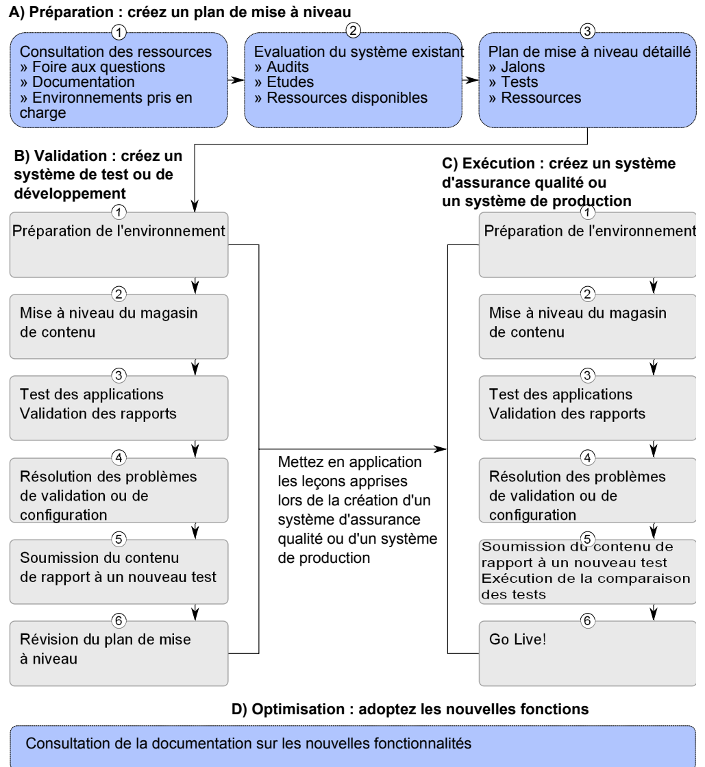
Figure 2. Processus de mise à niveau
