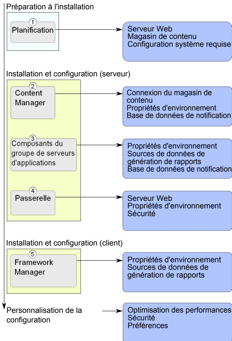
Figure 3. Flux de travaux du processus d'installation répartie
